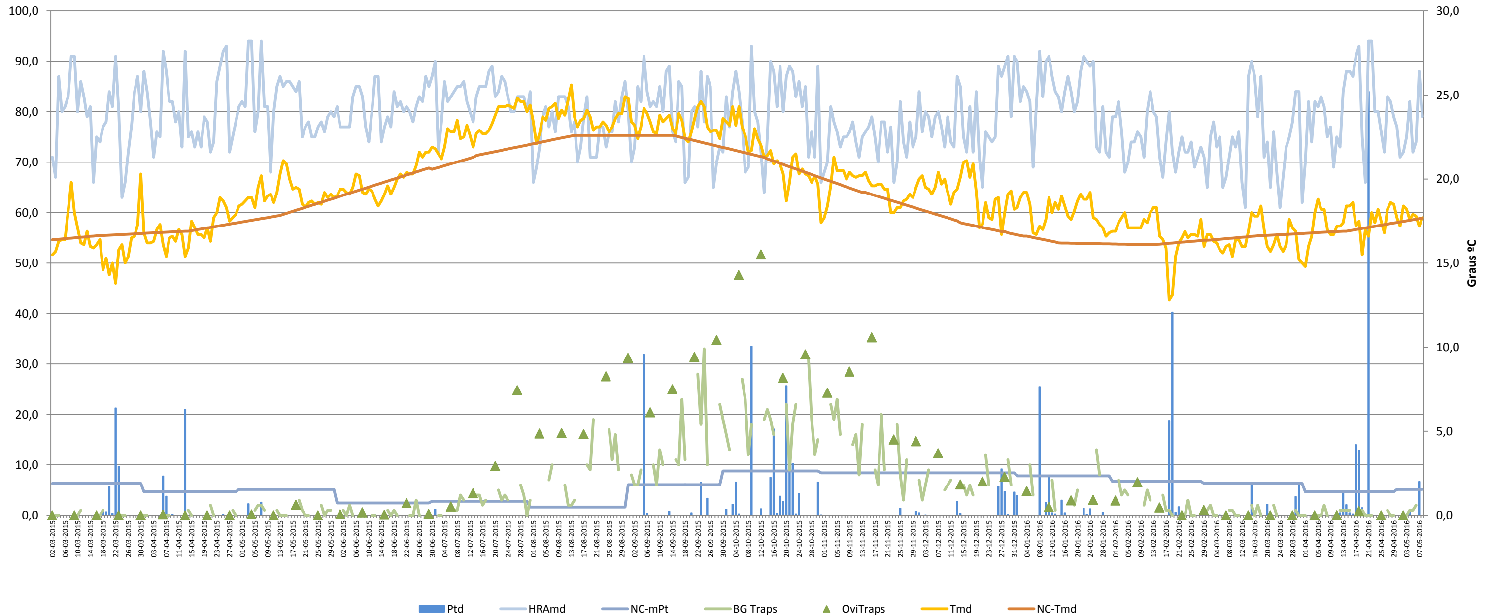
Gráfico com o cruzamento dos dados meteorológicos (precipitação total diária*, temperatura média diária* e humidade relativa do ar máxima diária*) e climáticos (normais climatológicas (1971-2000)*) com os dados entomológicos (nº mosquitos fêmea e nº ovos Aedes aegypti) desde a semana 10 de 2015 até à semana 18 de 2016
